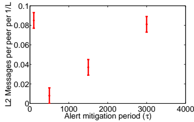
(d) Cost vs. \tau
